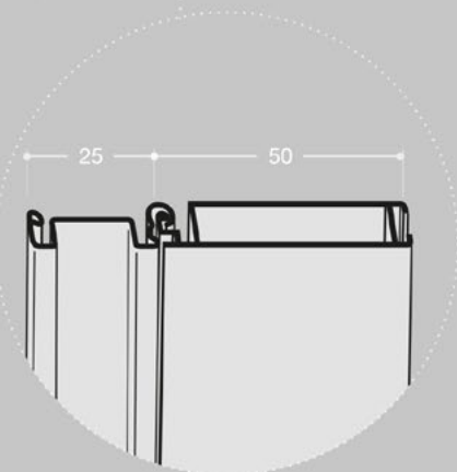
PROFIL MIT GRIFF cod. FBS7547 + FBS2010 ( Griff )
