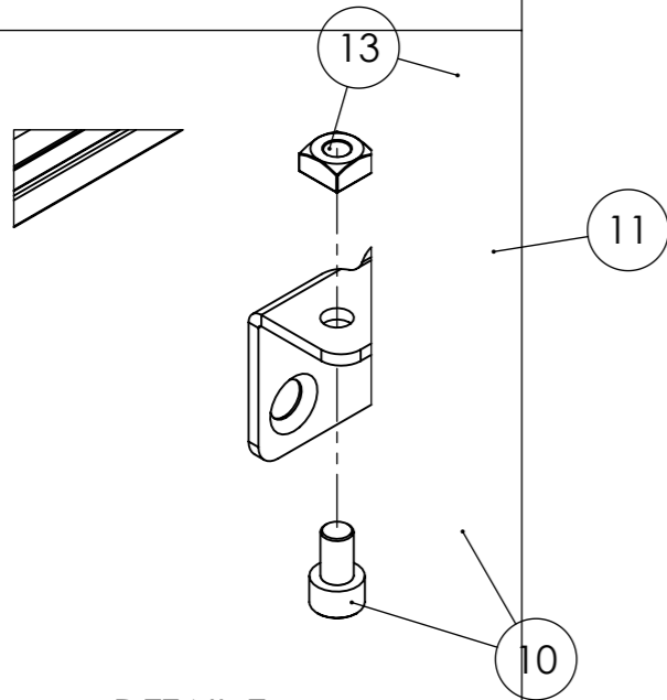
DETAIL E MABSTAB 2 : 3
